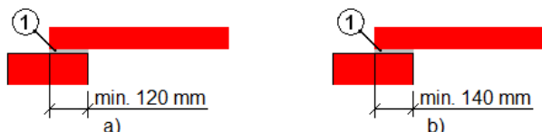
Obr. 1 Minimálna dĺžka uloženia keramického prekladu ATLAS 11,5
