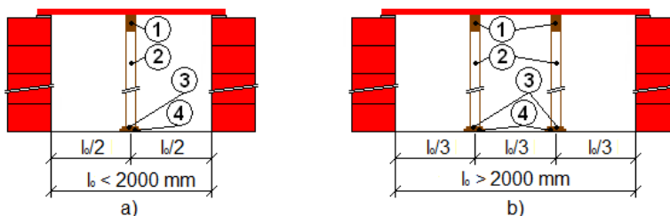
Obr. 2 Montážne pôdopretie keramických prekladov ATLAS 11,5
