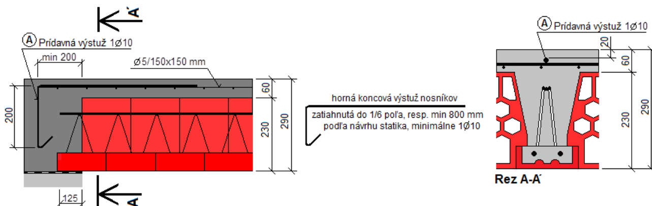
Obr. 18 Prídavná horná výstuž nad podperou pri nosníkoch dĺžky \geq 6000 mm, hrúbky 290 mm
