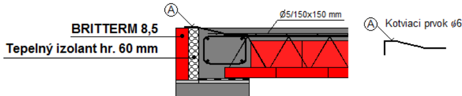
Obr. 22 Stratené debnenie vytvorené výrobkom BRITTERM 8,5 a tepelného izolantu
