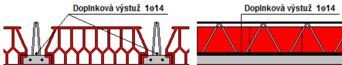
Obr. 19 Umiestnenie doplnkovej výstuže na nosníku
