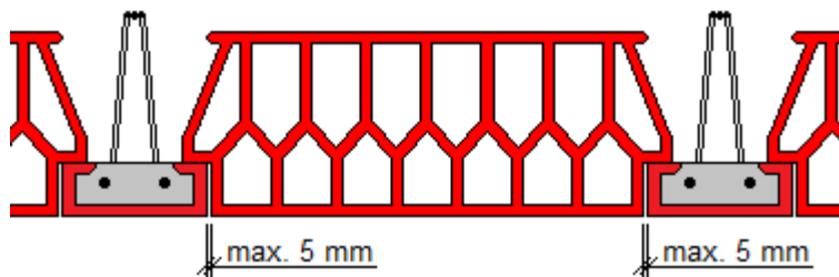
Obr. 7 Umiestnenie MIAKA medzi nosníkmi
