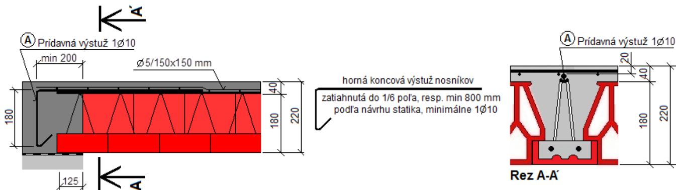
Obr. 16 Prídavná horná výstuž nad podporou pri nosníkoch dĺžky \geq 5000 mm, hrúbky 220 mm
