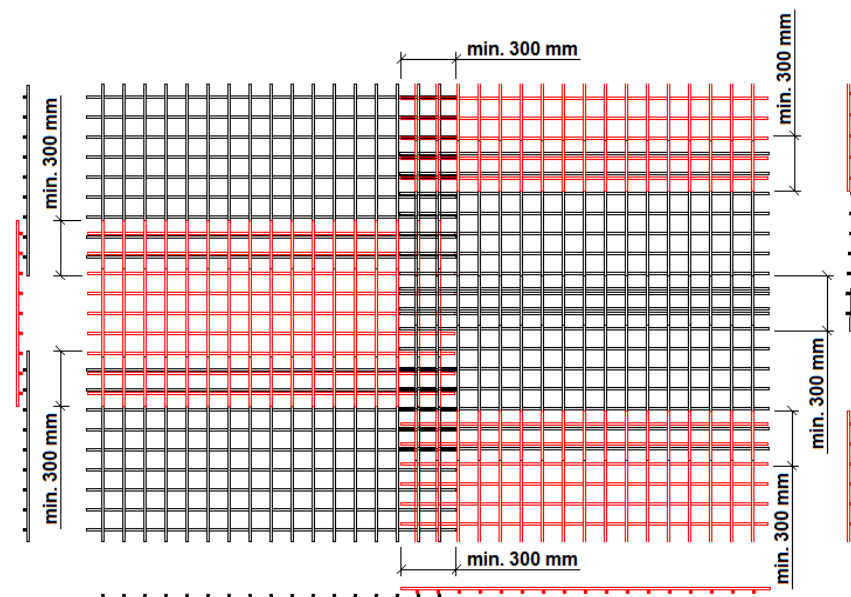
Obr. 14 Stykovanie zváraných sietí presahom
