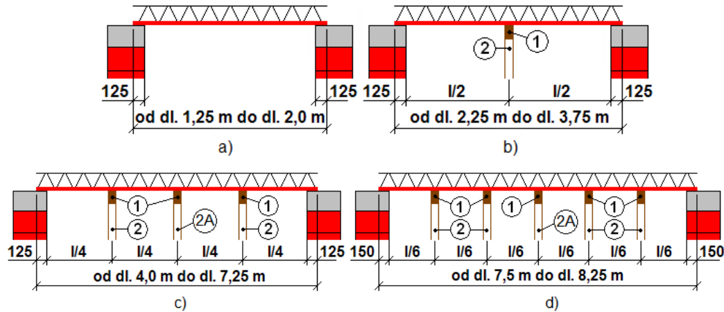
Obr. 8 Počet a umiestnenie stojok v rovine rovnobežnej s nosníkmi
