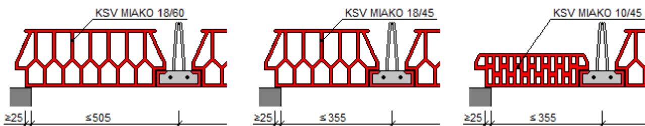
Obr. 12 Uloženie MIAKA na nosnú stenu
