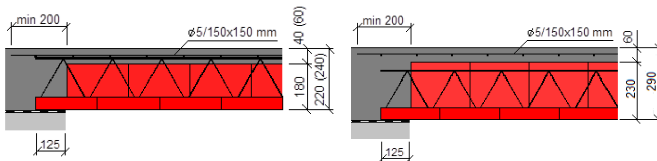
Obr. 15 Zatiahnutie zváraných sietí za líce podpery
