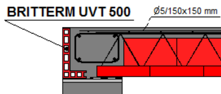
Obr. 23 Stratené debnenie vytvorené výrobkom BRITTERM UVT 500
