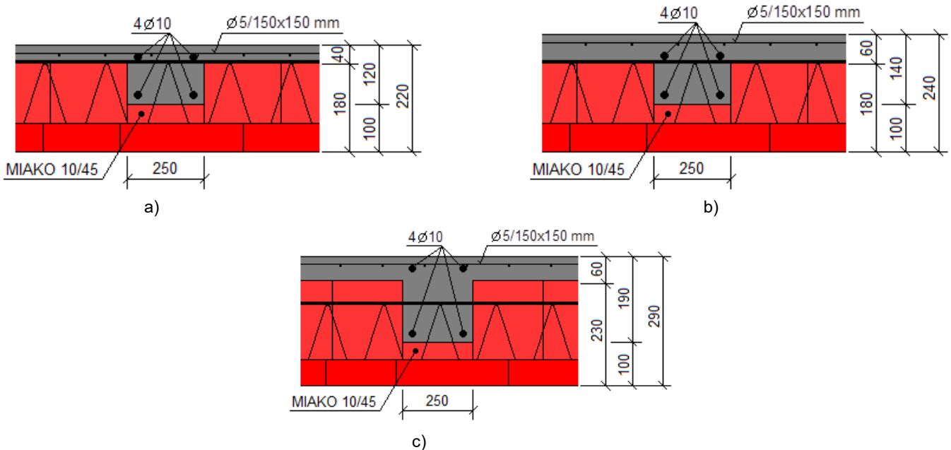
Obr. 21 Stučujúce rebro s použitím keramickej vložky MIAKO 10/45
