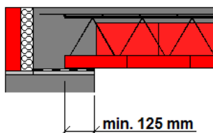
Obr. 5 Minimálne uloženie stropných nosníkov BRITTERM
