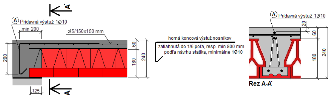
Obr. 17 Prídavná horná výstuž nad podperou pri nosníkoch dĺžky \geq 6000 mm, hrúbky 240 mm
