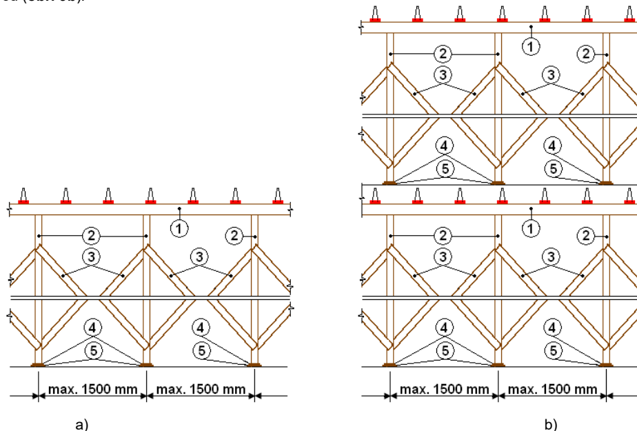
Obr. 9 Umiestnenie montážnych stojok v rovine kolmej na nosníky
