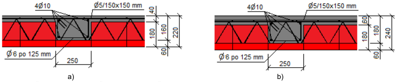
Obr. 20 Stučujúce rebro bez použitia keramickej vložky MIAKO 10/45
