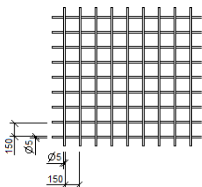
Obr. 13 Zváraná sieťovina \text{Ø}5/150 \times 150 mm
