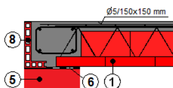
Obr. 28 Stratené debnenie vytvorené výrobkom BRITTERM UVT 500
