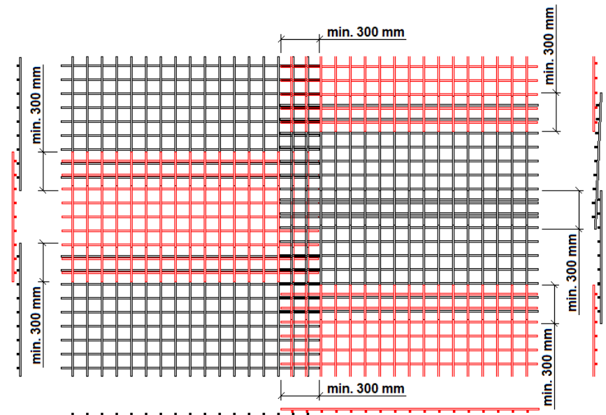
Obr. 17 Stykovanie zväraných sietí presahom
