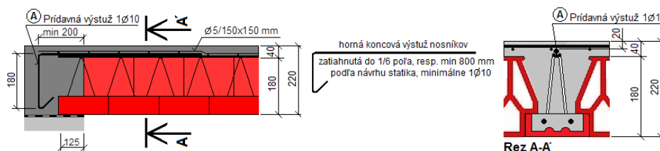
Obr. 21 Prídavná horná výstuž nad podporou pri nosníkoch dĺžky \geq 5000 mm, hrúbky 220 mm
