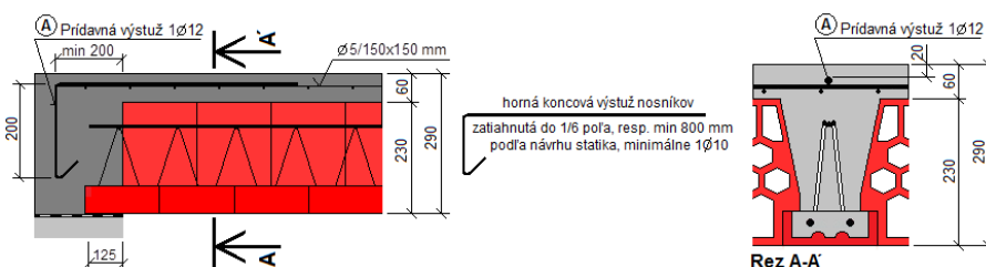
Obr. 23 Prídavná horná výstuž nad podporou pri nosníkoch dĺžky \geq 6000 mm, hrúbky 290 mm
