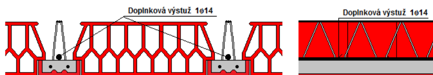
Obr. 24 Umiestnenie doplnkovej výstuže na nosníku
