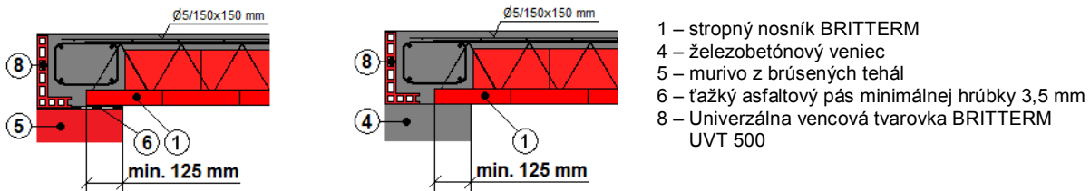
Obr. 6 Minimálne uloženie stropných nosníkov BRITTERM
