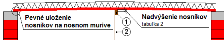
Obr. 13 Pevné uloženie nosníkov na nosnom murive
