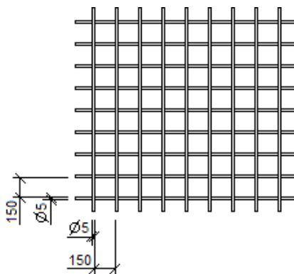
Obr. 16 Zváraná sieťovina \varnothing 5/150 \times 150 mm
