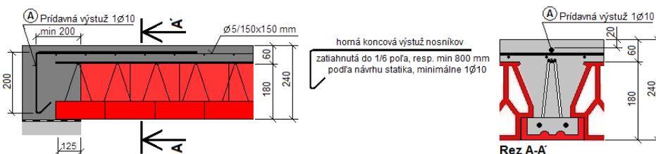
Obr. 22 Prídavná horná výstuž nad podporou pri nosníkoch dĺžky \geq 6000 mm, hrúbky 240 mm
