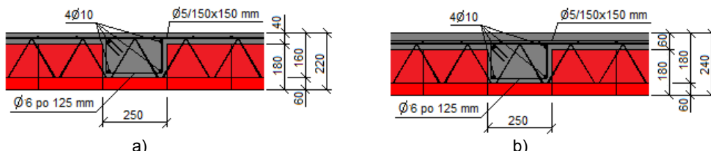
Obr. 25 Stužujúce rebro bez použitia keramickej vložky MIAKO 10/45
