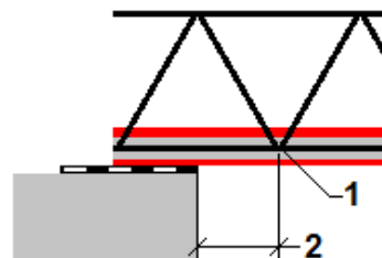
Obr. 31 Zásada pri skracovaní nosníka
