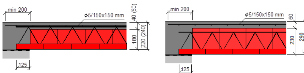
Obr. 18 Zatiahnutie zväraných sietí za líce podpery
