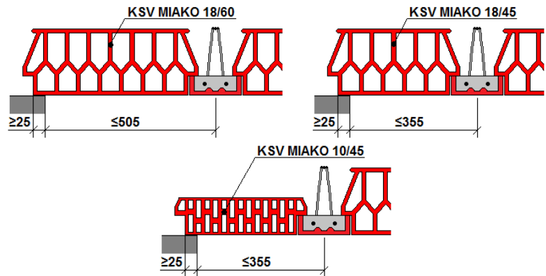
Obr. 15 Uloženie MIAKA na nosnú stenu
