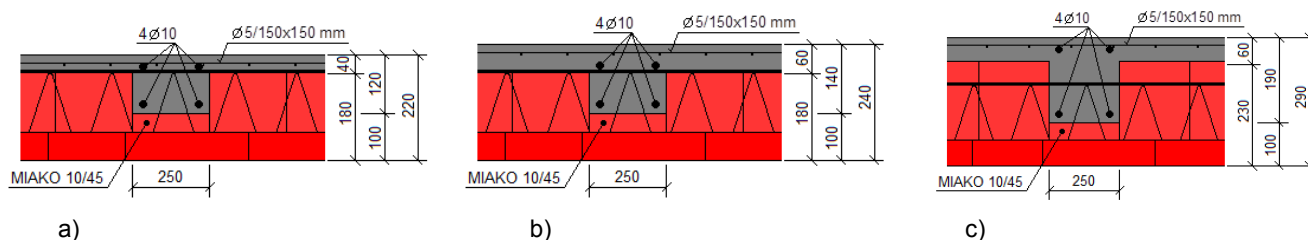
Obr. 26 Stužujúce rebro s použitím keramickej vložky MIAKO 10/45
