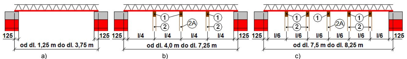
1 – drevený hranol
