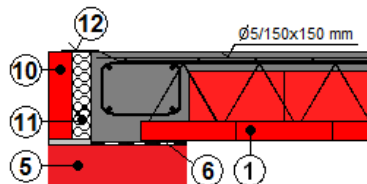
Obr. 27 Stratené debnenie vytvorené výrobkom BRITTERM 8,5 a tepelného izolantu
